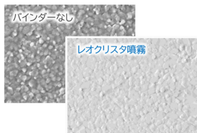
レオクリスタを噴霧した場合は焼結体が 高密度化し、表面が平滑になる
