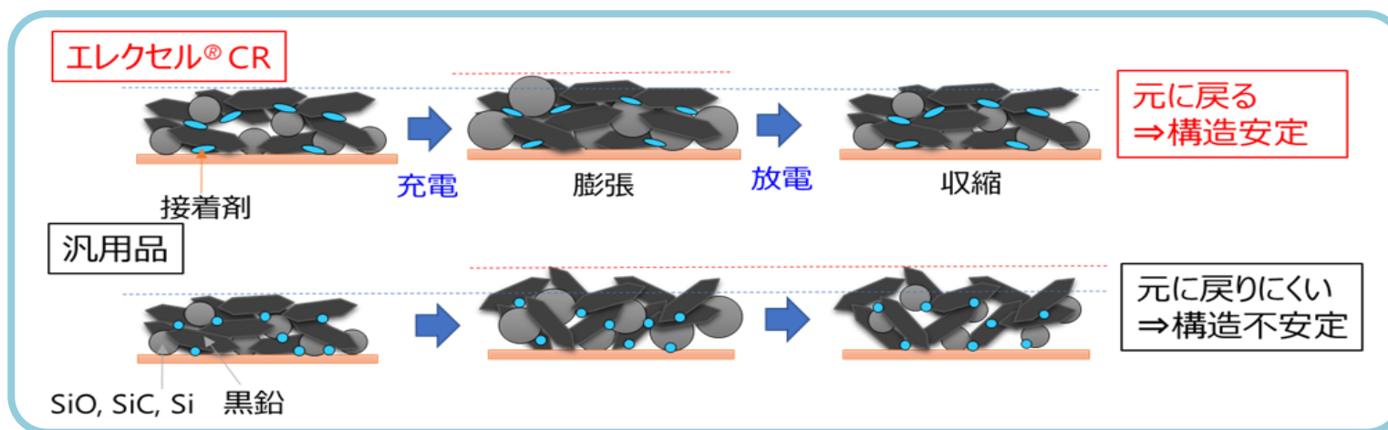
充放電における開発品「Elexcel CR」と汎用品の電極の構造変化のイメージ図
