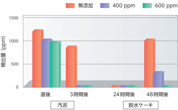
■ 硫化水素の消臭効果
