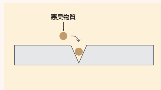
細孔内への物理吸着
