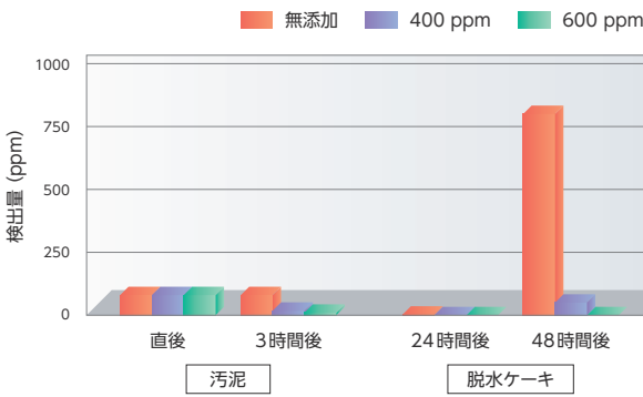
■ メチルメルカプタンの消臭効果
