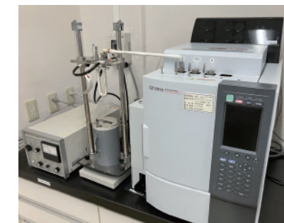
ガスクロマトグラフィー（GC）
