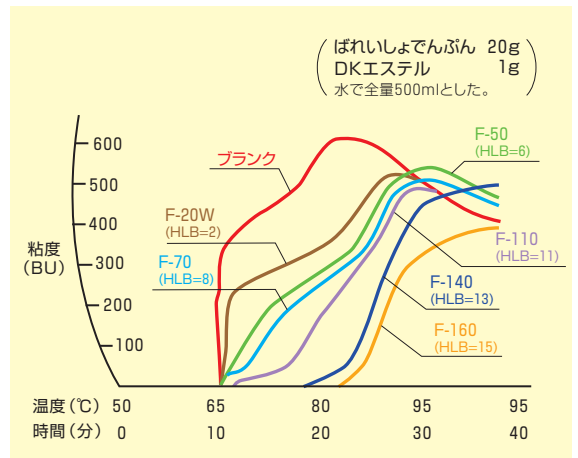
図2 DKエステルのでんぷんとの相互作用※
