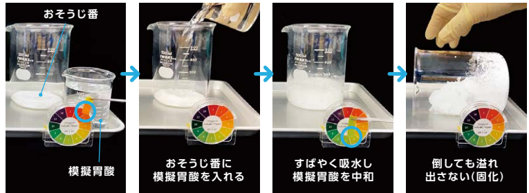
図2 模擬胃酸(pH2)条件下における吸水・中和・固化の様子
